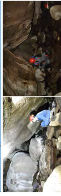
Sistema de cuevas de A Cunchosa
